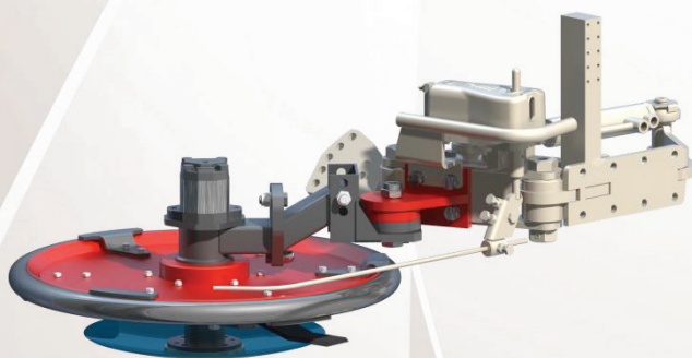
Tincia erba flottante Floating slasher
